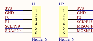
Micro:bit GPIO
